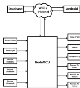
Gambar 5. Desain diagram sistem
